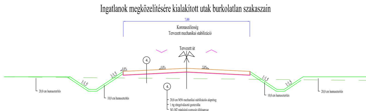
A Nyugati elkerülő út szervizútjainak tervezett mintakeresztmetszévényei Tervező: Cívis Komplex Mérnök Kft. (4030 Debrecen, Gizella u 13/D.)
