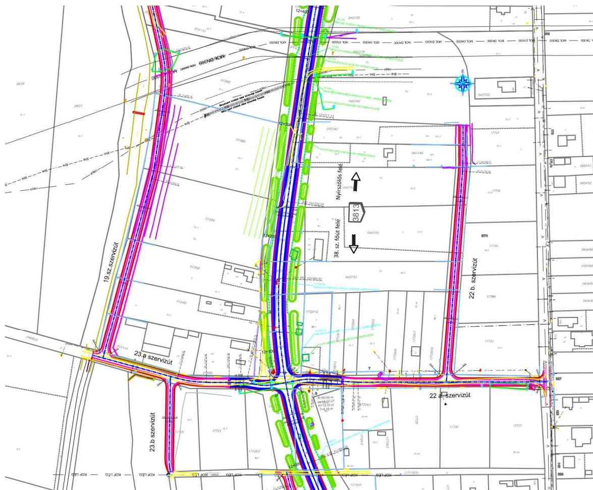
A Nyugati elkerülő út és szervizutjainak építési helyszínrajza (részlet) Tervező: Cívis Komplex Mérnök Kft. (4030 Debrecen, Gizella u 13/D.)
