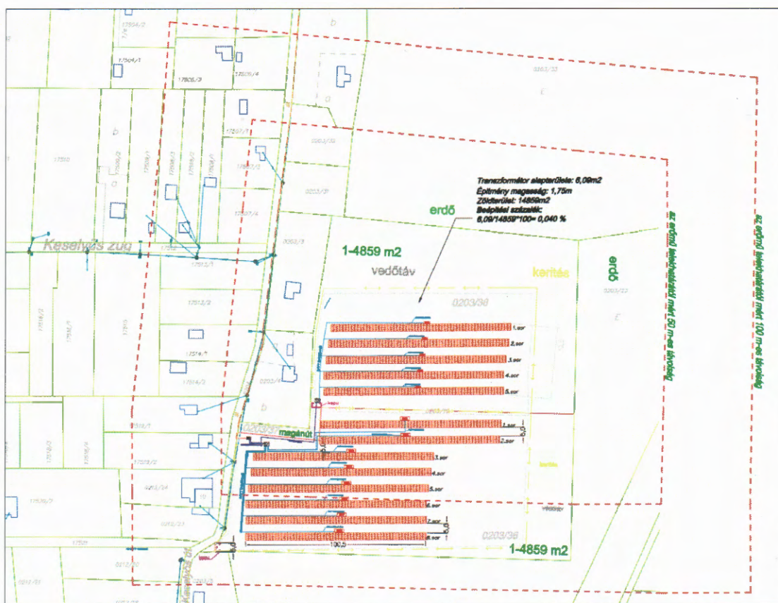
Beépítési tanulmányterv a 2. sz. kiserőműhöz
